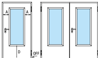
Verglasung Bild 3
