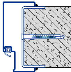
Umfassungszarge B73 Schweißmontage D Typ 2
