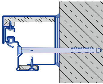
Blockzarge 2-schalig Dübelmontage durch die Zargenlaibung E Typ 2
