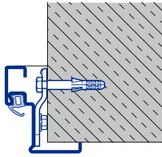
Eckzarge Dübelmontage verdeckt A Typ 2
