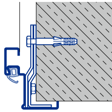
Eckzarge Dübelmontage in der Laibung A Typ 2 / A Typ 3
