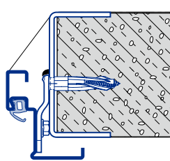
Eckzarge Schweißmontage A Typ 2 / A Typ 3
