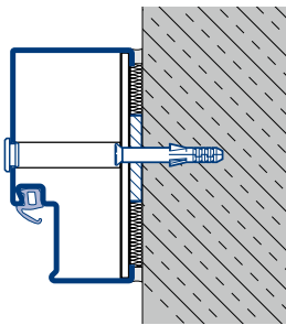
Blockzarge Dübelmontage durch die Zargenlaibung E Typ 1
