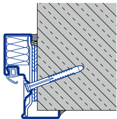
DryFix Zarge Diagonalbefestigung B Typ 1
