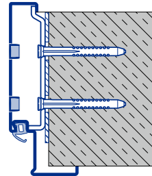
Umfassungszarge Dübelmontage durch die Zargen- laibung ab MW 205 mm D Typ 1
