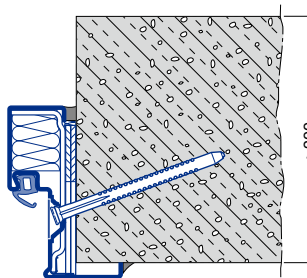
DryFix Zarge Diagonalfestigung B Typ 1
