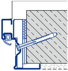
Eckzarge Diagonalfestigung A Typ 1
