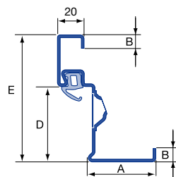
Eckzarge Diagonalbefestigung
