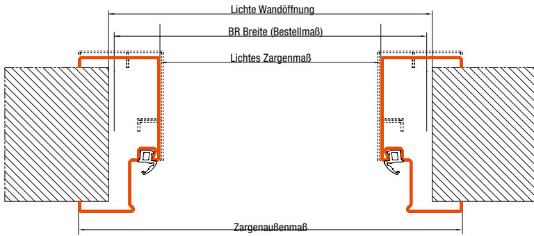
3-seitig umlaufende Zarge (Türen) BR Breite BR Höhe
