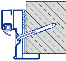
Eckzarge Diagonalbefestigung A Typ 1
