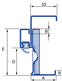
Eckzarge mit Ergänzungszarge Vario B53
