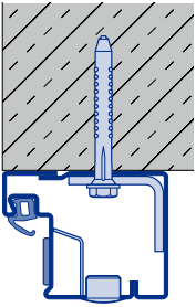
Blockzarge für den Einbau vor die Wand E Typ 3
