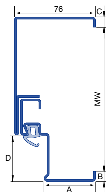
Umfassungszarge 2-schalig
