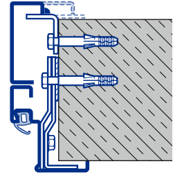
Eck- und Ergänzungszarge Dübelmontage C Typ 3
