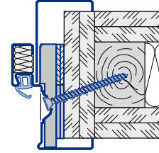
Eckzarge mit Ergänzungszarge Vario B53 Diagonalfestigung C Typ 1
