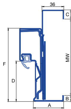
DryFix Zarge mit Ergänzungszarge Vario B36 bis RC 2
