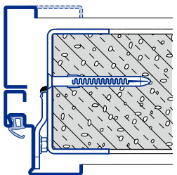
Eck- und Ergänzungszarge Schweißmontage C Typ 3
