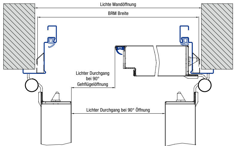
2-flügelige Tür
