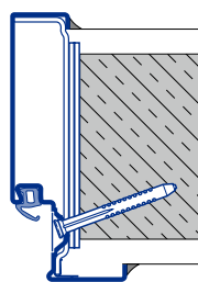
Umfassungszarge Diagonalfestigung bis MW 175 D Typ 1
