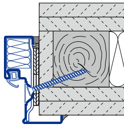
DryFix Zarge Diagonalfestigung B Typ 1
