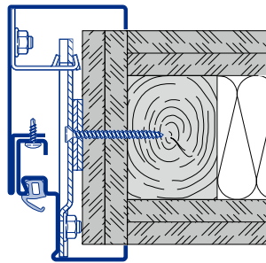
Umfassungszarge 2-schalig (Zargenspiegel 76 mm) Ständerwände F90 B D Typ 3
