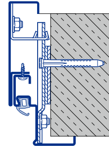
Umfassungszarge 2-schalig Zargenspiegel 33 mm D Typ 3
