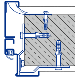
Eckzarge mit Ergänzungszarge Dübelmontage C Typ 3
