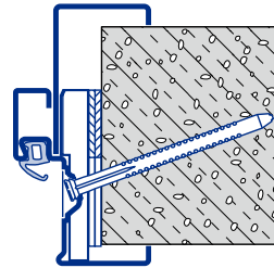
Eckzarge mit Ergänzungszarge Vario B53 Diagonalfestigung C Typ 1
