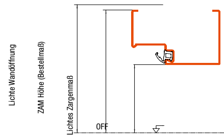
4-seitig umlaufende Zarge (Tür) ZAM Breite ZAM Höhe
