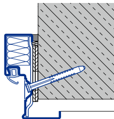
DryFix Zarge Diagonalfestigung B Typ 1
