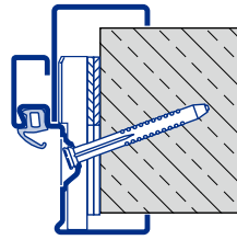
Eckzarge mit Ergänzungszarge Vario B53 Diagonalbefestigung C Typ 1
