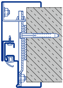
Umfassungszarge 2-schalig Zargenspiegel 76 mm D Typ 3
