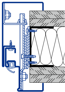
Umfassungszarge 2-schalig (Zargenspiegel 76 mm) Ständerwände F90 A D Typ 3
