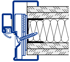
Universal-Eckzarge mit Ergänzungszarge Vario B53 Diagonalfestigung C Typ 1
