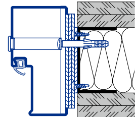
Blockzarge Dübelmontage durch die Zargenlaibung E Typ 1
