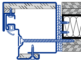
Blockzarge 2-schalig Dübelmontage durch die Zargenlaibung E Typ 2
