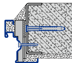
Eckzarge Dübelmontage A Typ 1
