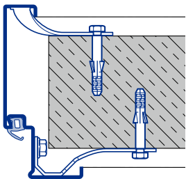
Umfassungszarge Dübelmontage D Typ 1
