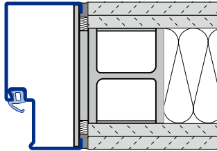
Blockzarge Schweißmontage E Typ 1
