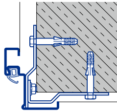
Eckzarge Montage über Mauereck A Typ 2 / A Typ 3
