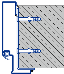
Umfassungszarge Dübel- / Schweißmontage D Typ 1
