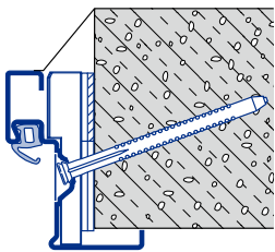
Eckzarge Diagonalfestigung A Typ 1
