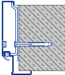
Umfassungszarge Dübelmontage durch die Zargenlaibung bis MW 204 mm D Typ 1
