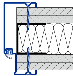
Umfassungszarge B73 für Ständerwände Schraubmontage C Typ 4
