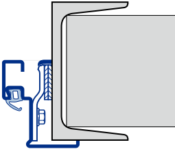
Eckzarge Schweißmontage A Typ 3
