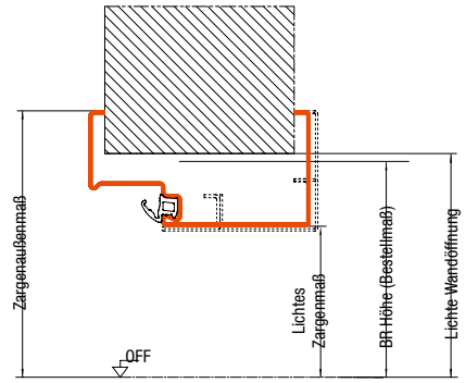
4-seitig umlaufende Zarge (Tür) BR Breite BR Höhe
