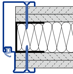
Umfassungszarge B73 für Ständerwände Schraubmontage C Typ 4
